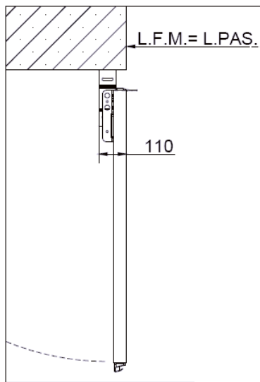
INGOMBRO 1 ANTA OLTRE LUCE 90° E 180°
