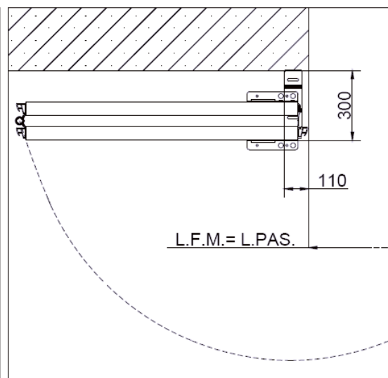
INGOMBRO 2 ANTE OLTRE LUCE 180°
