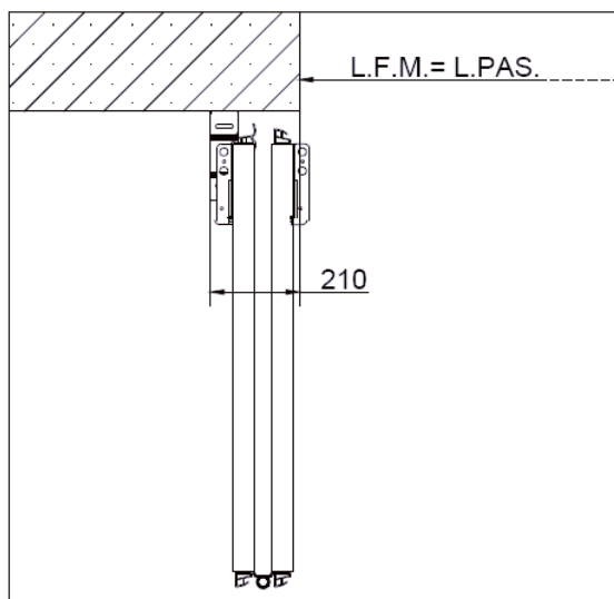
INGOMBRO 2 ANTE OLTRE LUCE 90°
